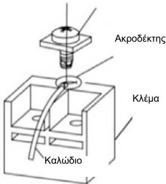
Βίδα με ροδέλα
