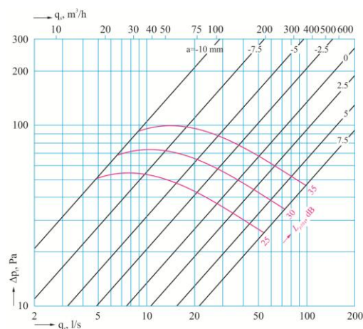
DVS-P 150 mm
