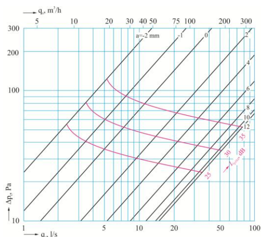
DVS-P 100 mm
