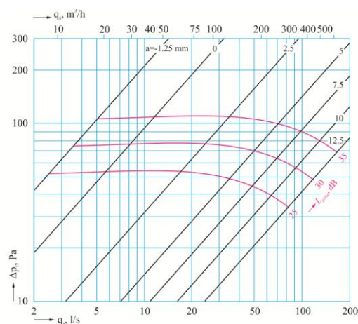
DVS-P 200 mm
