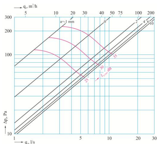
DVS-P 080 mm
